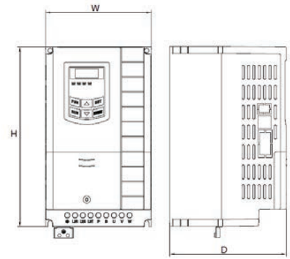
Frame 3 (IP20)
